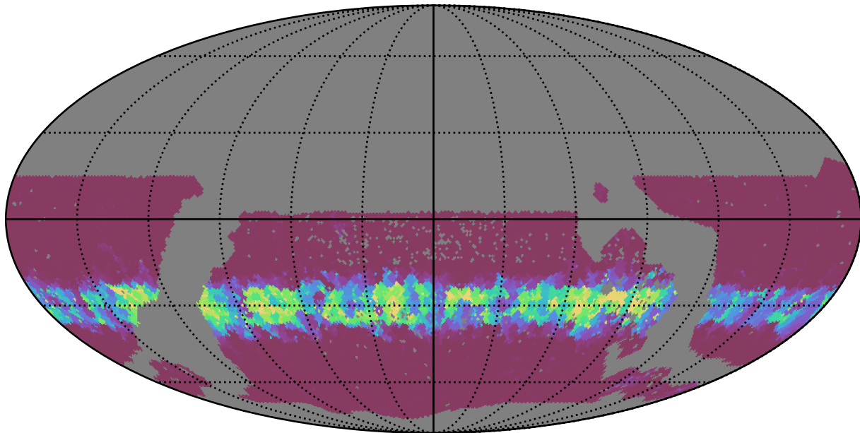
mw_roll_bulge_v3.3_10yrs WFD u band: Min normairmass
