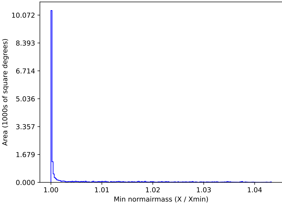
mw_roll_bulge_v3.3_10yrs WFD u band: Min normairmass
