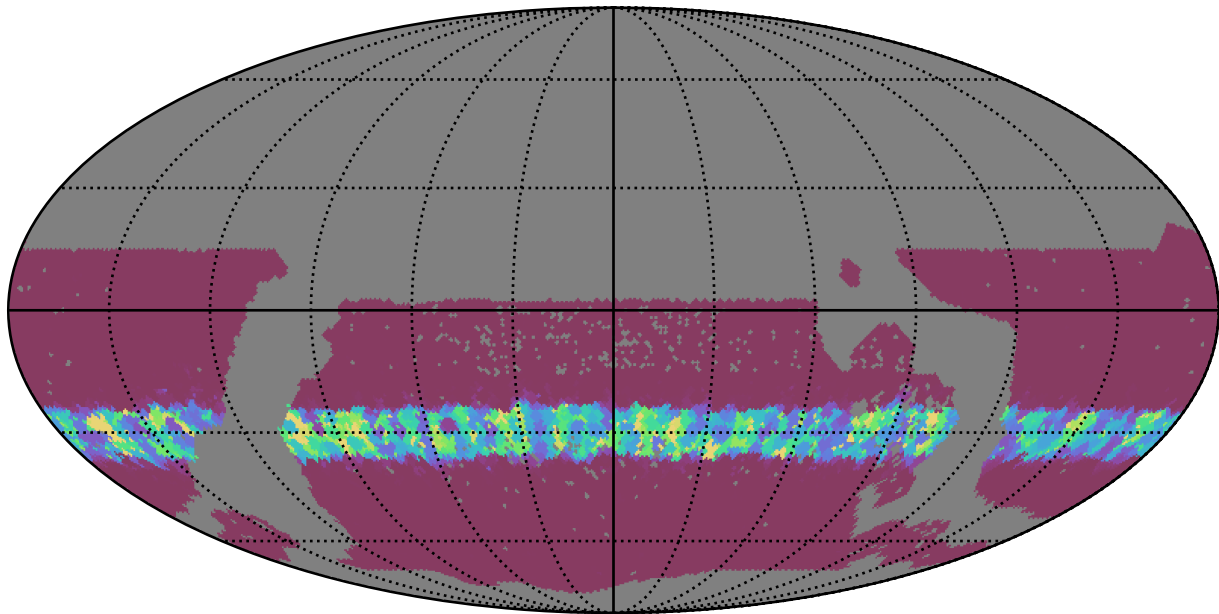
mw_roll_bulge_v3.3_10yrs WFD r band: Min normairmass
