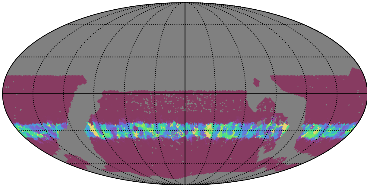
mw_roll_bulge_v3.3_10yrs WFD i band: Min normairmass
