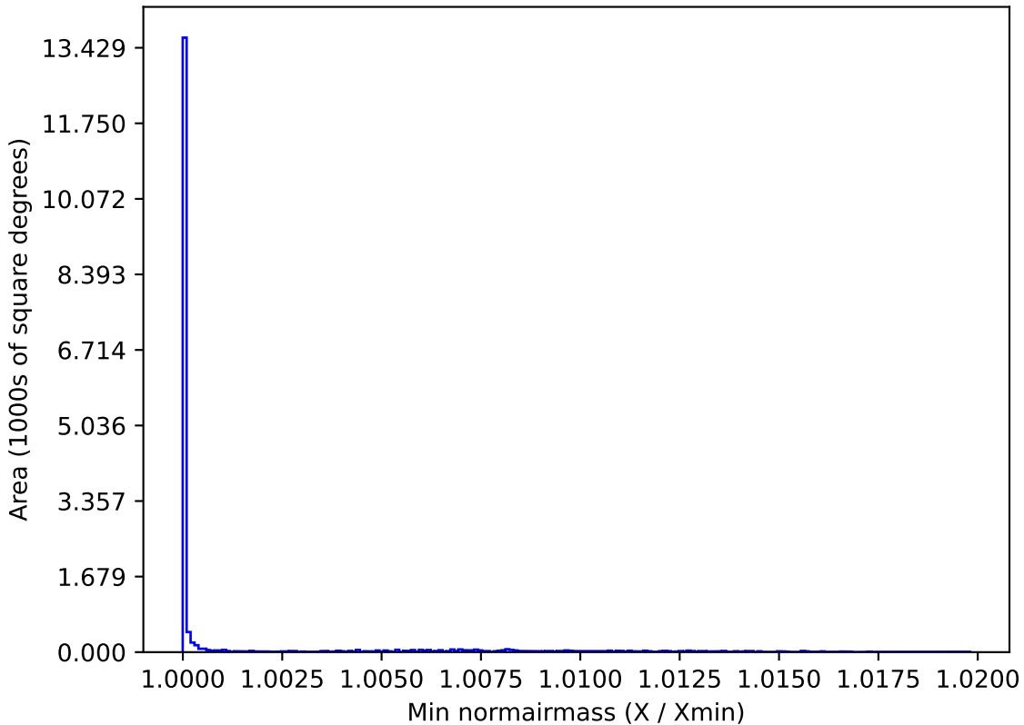
mw_roll_bulge_v3.3_10yrs WFD i band: Min normairmass
