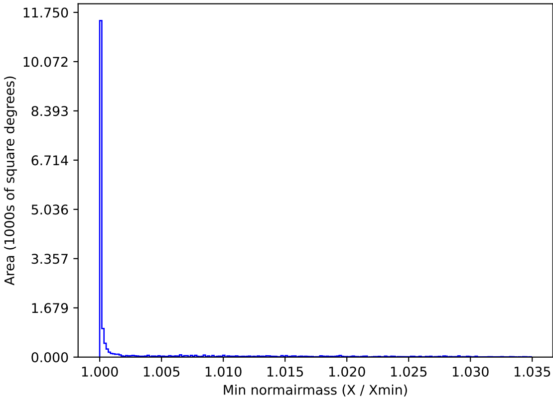
mw_roll_bulge_v3.3_10yrs WFD g band: Min normairmass
