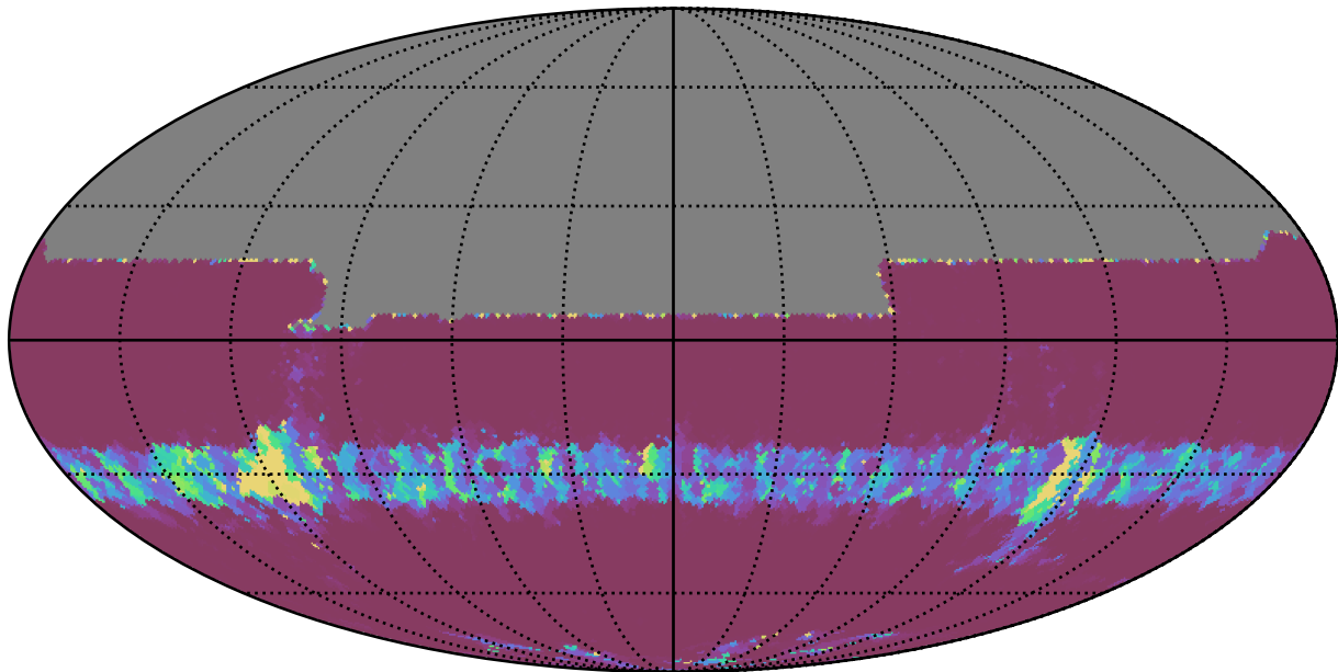
mw_roll_bulge_v3.3_10yrs All sky y band: Min normairmass
