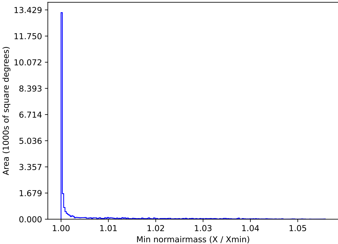
mw_roll_bulge_v3.3_10yrs All sky u band: Min normairmass
