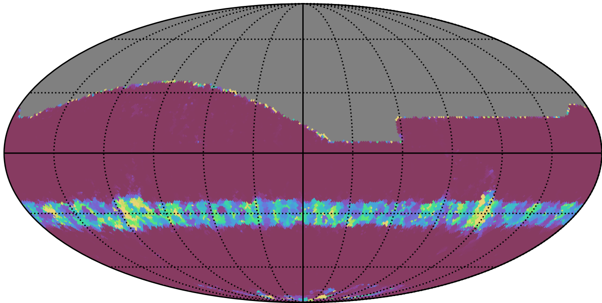
mw_roll_bulge_v3.3_10yrs All sky r band: Min normairmass
