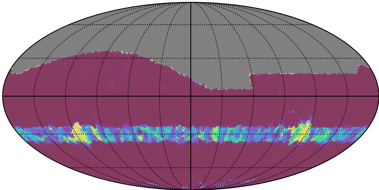
mw_roll_bulge_v3.3_10yrs All sky i band: Min normairmass
