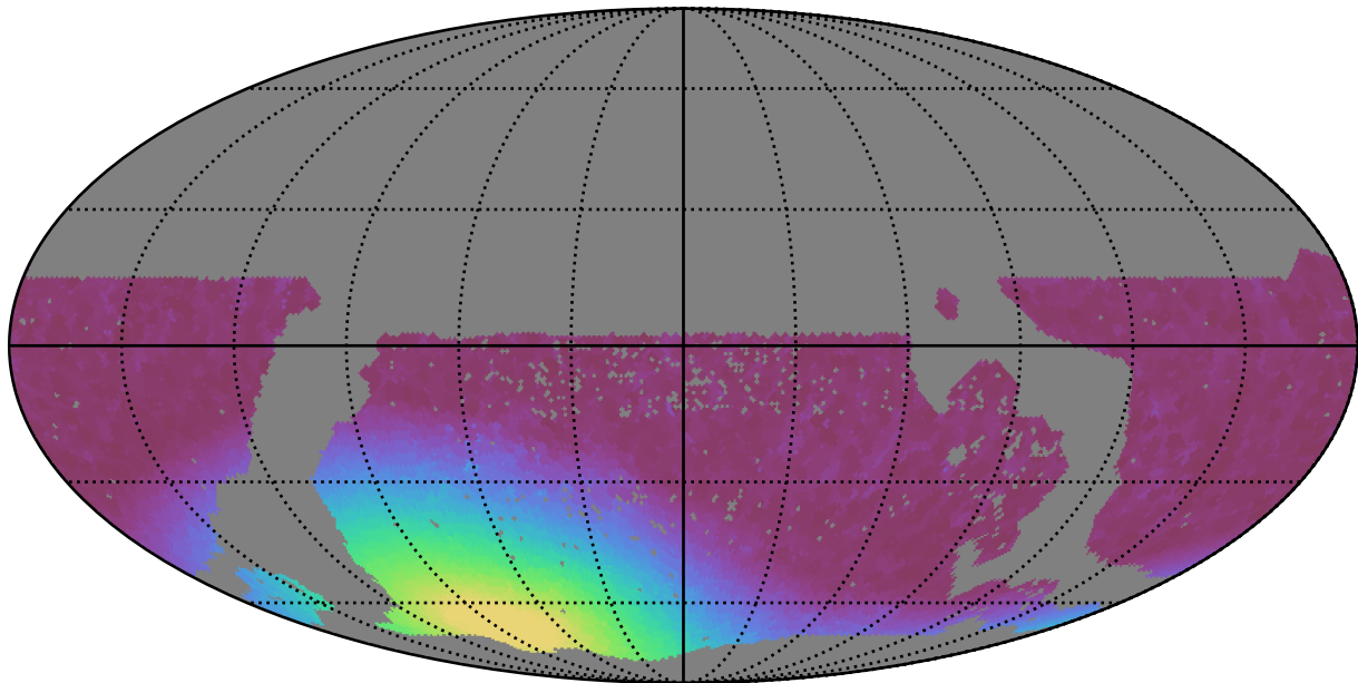
mw_roll_bulge_v3.3_10yrs WFD i band: Min moonDistance
