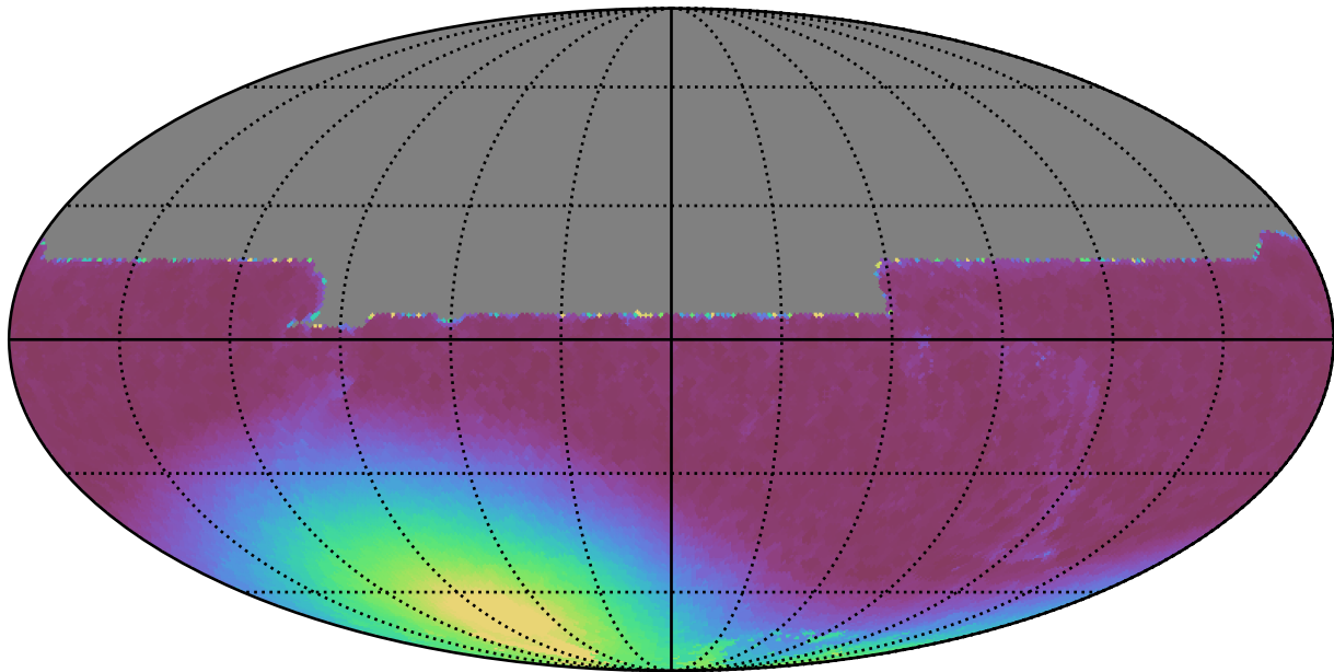
mw_roll_bulge_v3.3_10yrs All sky y band: Min moonDistance
