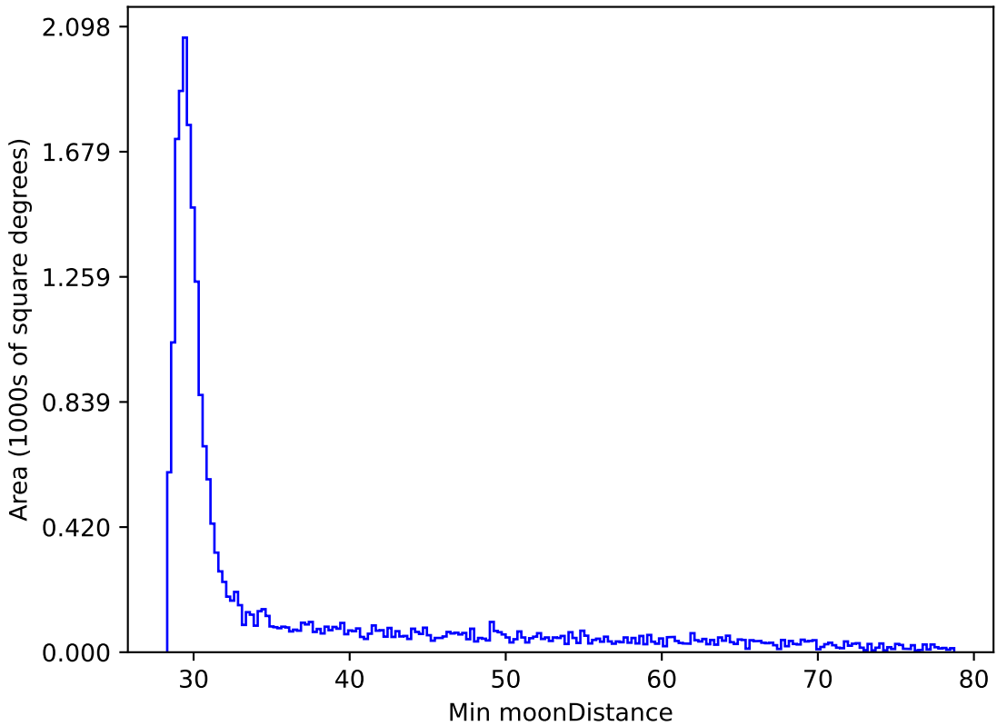
mw_roll_bulge_v3.3_10yrs All sky y band: Min moonDistance
