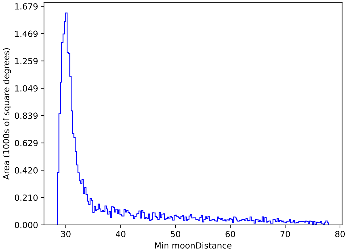
mw_roll_bulge_v3.3_10yrs All sky i band: Min moonDistance
