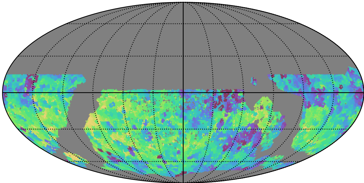
mw_roll_bulge_v3.3_10yrs WFD y band: Min fiveSigmaDepth
