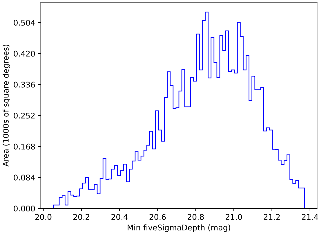
mw_roll_bulge_v3.3_10yrs WFD y band: Min fiveSigmaDepth
