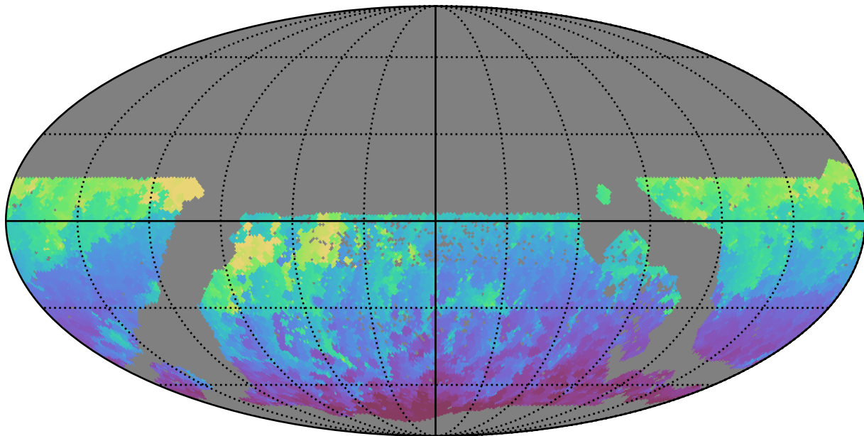
mw_roll_bulge_v3.3_10yrs WFD z band: Min HA
