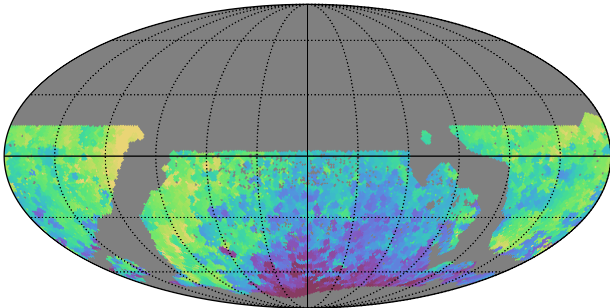
mw_roll_bulge_v3.3_10yrs WFD y band: Min HA
