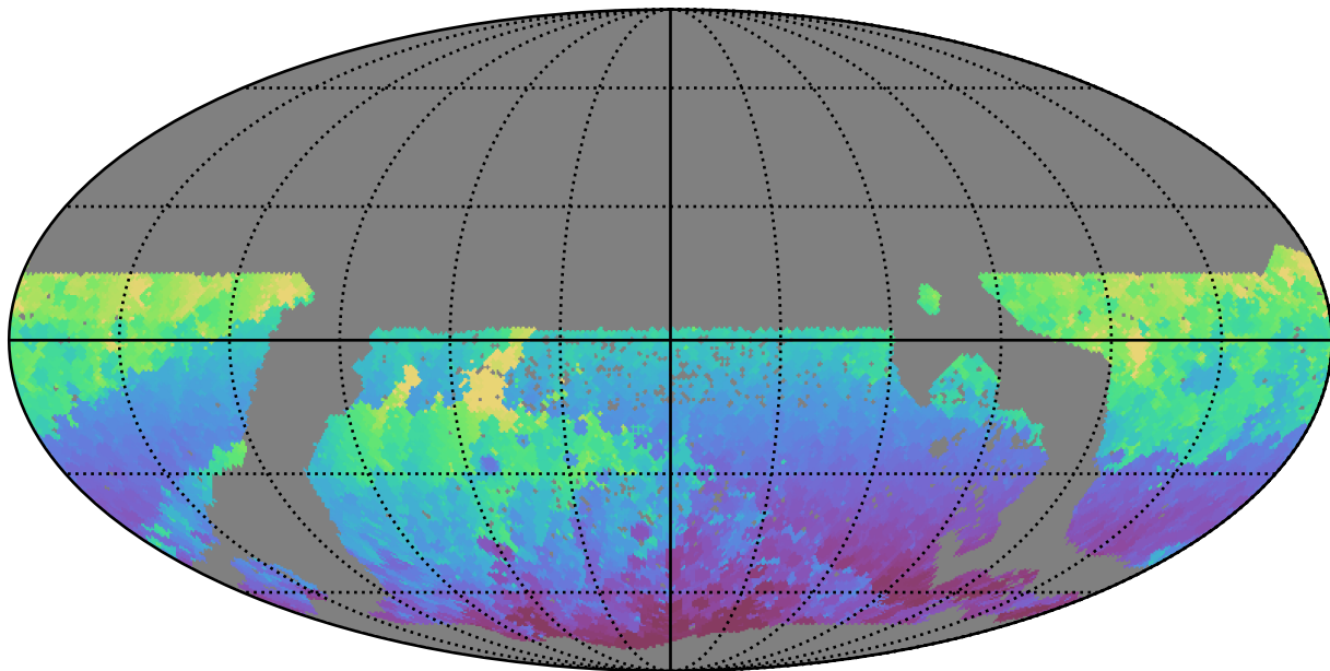
mw_roll_bulge_v3.3_10yrs WFD r band: Min HA
