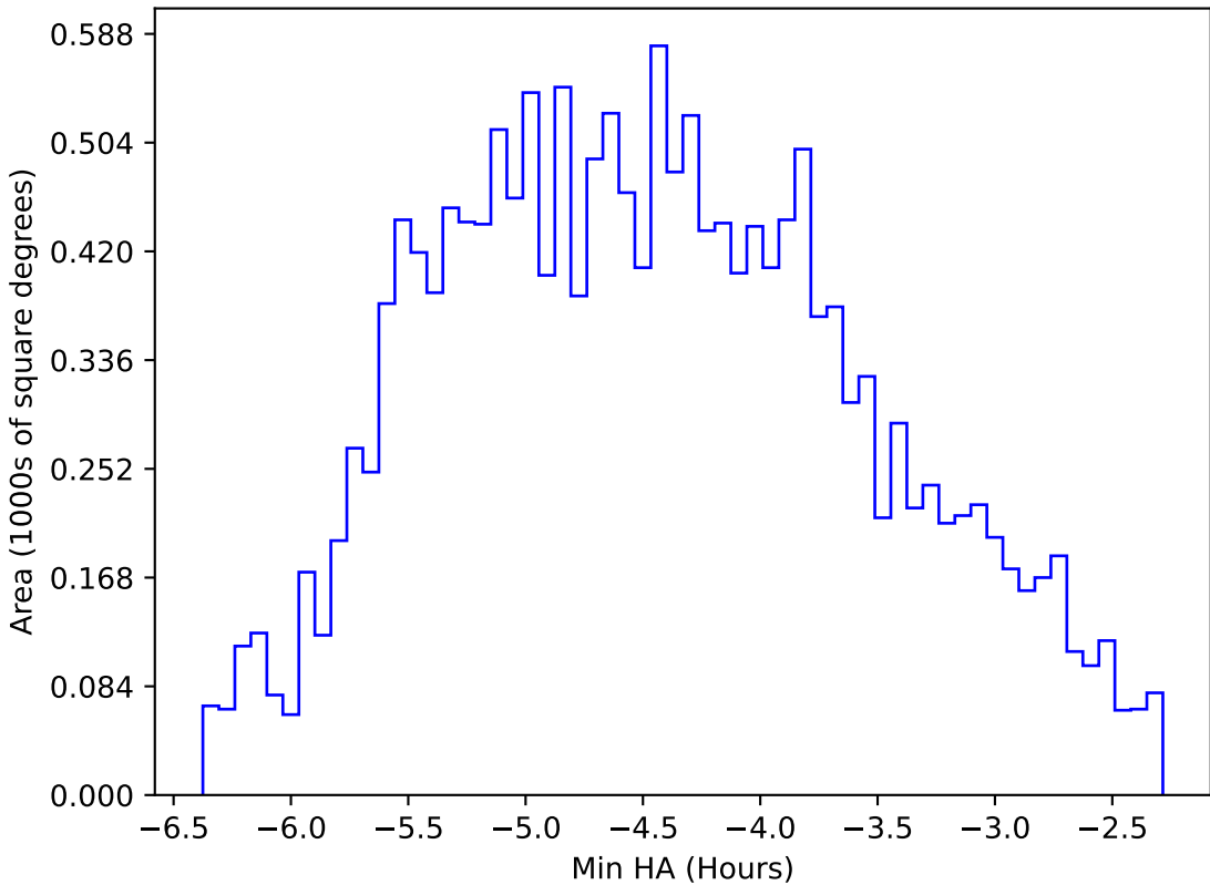
mw_roll_bulge_v3.3_10yrs WFD r band: Min HA
