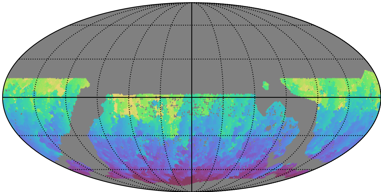
mw_roll_bulge_v3.3_10yrs WFD g band: Min HA
