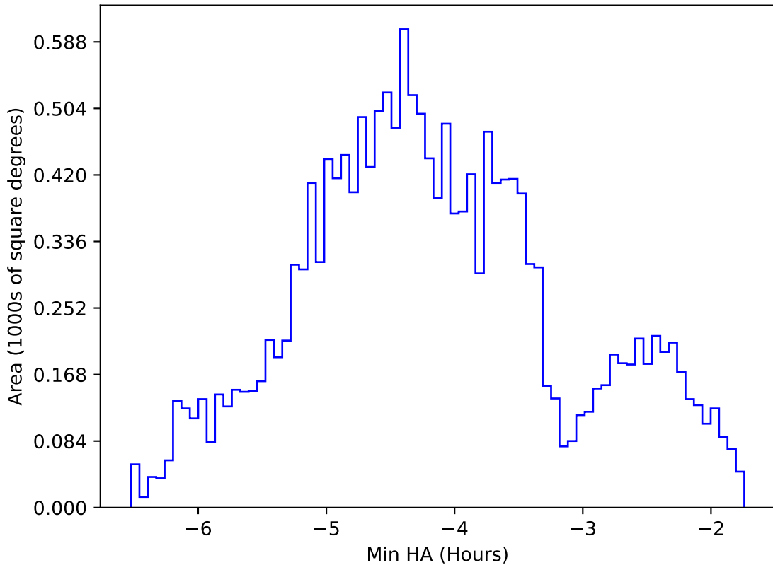
mw_roll_bulge_v3.3_10yrs WFD g band: Min HA
