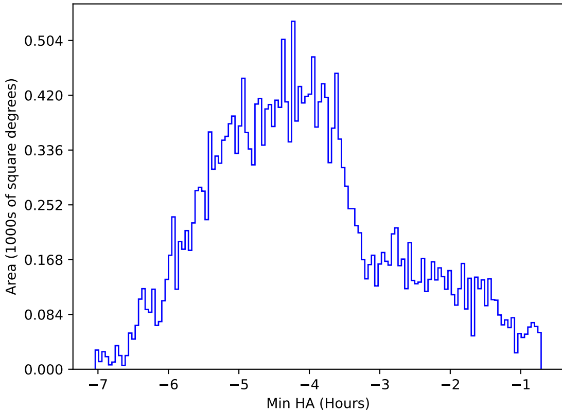
mw_roll_bulge_v3.3_10yrs All sky z band: Min HA
