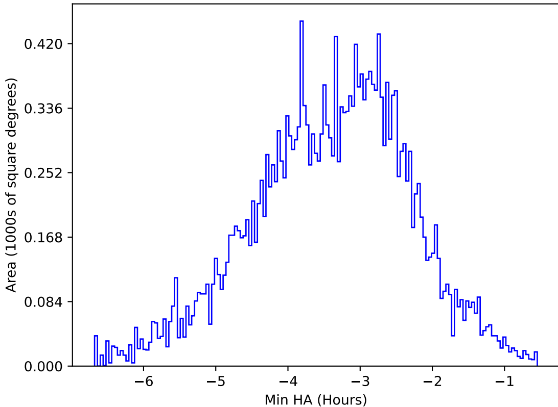
mw_roll_bulge_v3.3_10yrs All sky y band: Min HA
