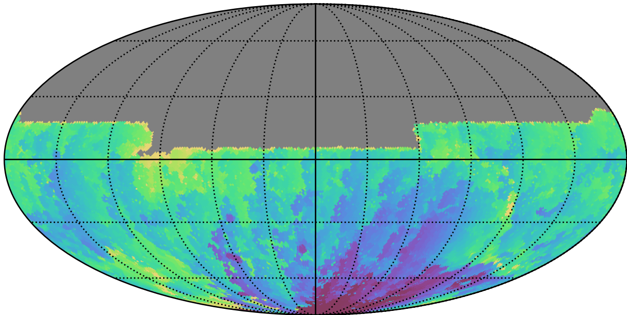
mw_roll_bulge_v3.3_10yrs All sky u band: Min HA
