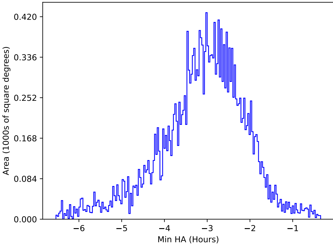
mw_roll_bulge_v3.3_10yrs All sky u band: Min HA
