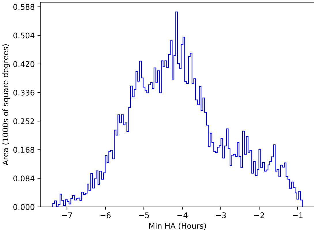
mw_roll_bulge_v3.3_10yrs All sky i band: Min HA
