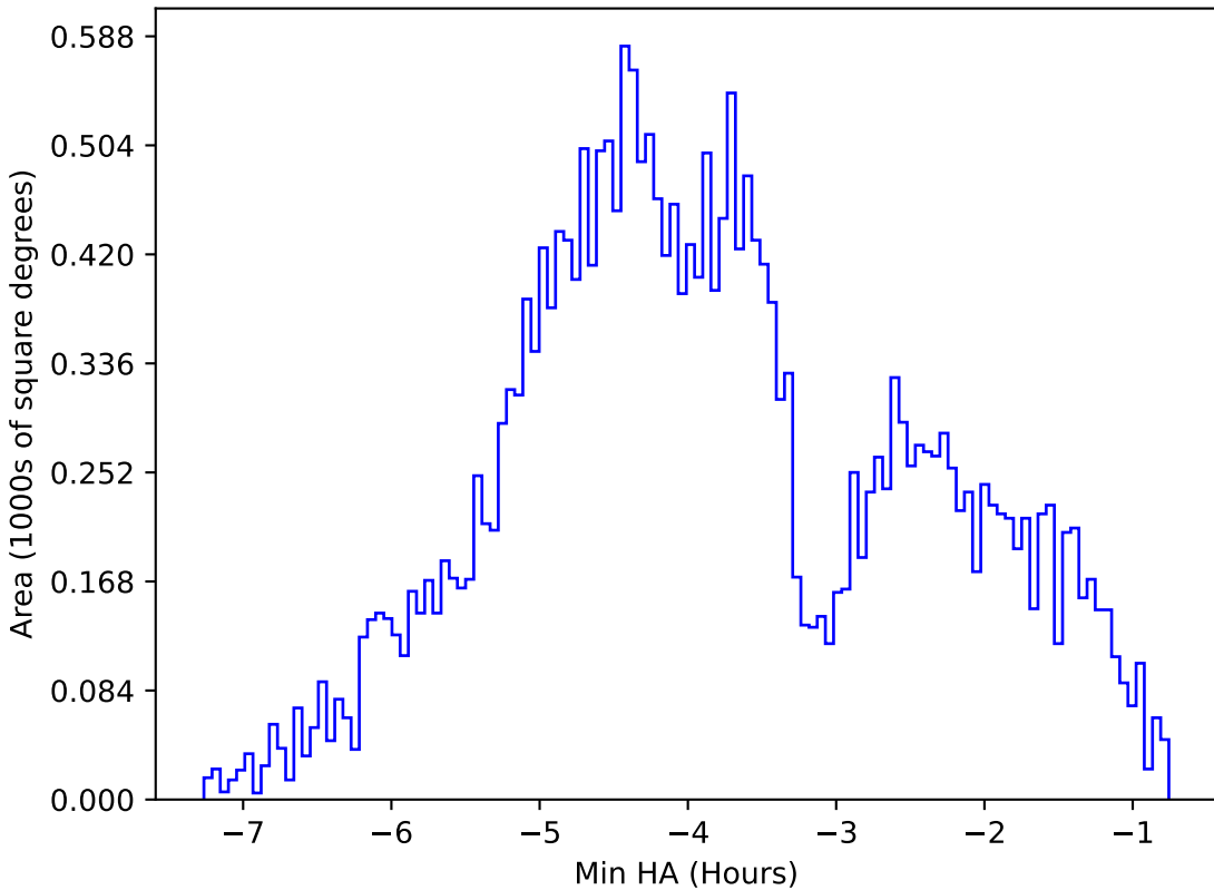
mw_roll_bulge_v3.3_10yrs All sky g band: Min HA
