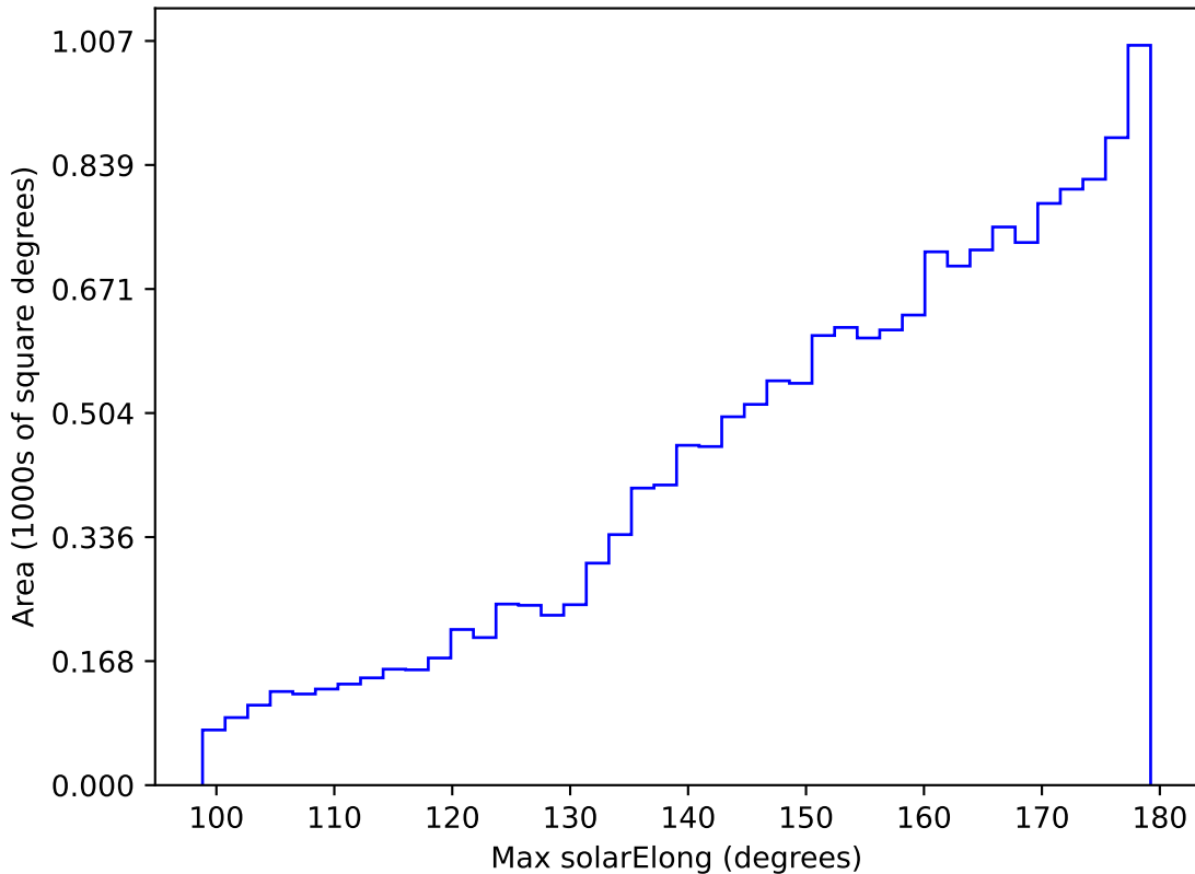
mw_roll_bulge_v3.3_10yrs WFD y band: Max solarElong
