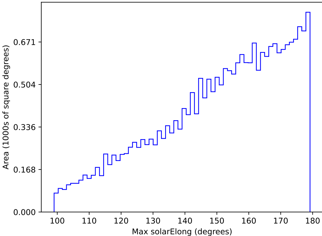
mw_roll_bulge_v3.3_10yrs All sky y band: Max solarElong
