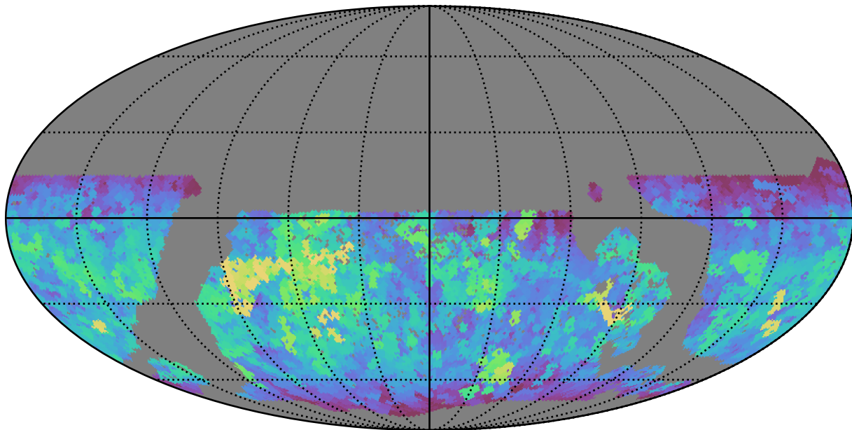
mw_roll_bulge_v3.3_10yrs WFD z band: Max saturation_mag
