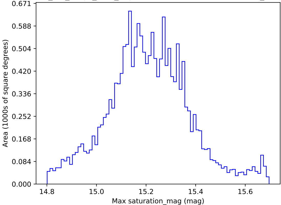
mw_roll_bulge_v3.3_10yrs WFD z band: Max saturation_mag
