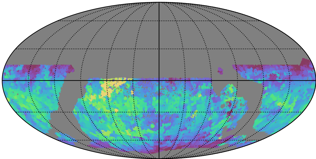
mw_roll_bulge_v3.3_10yrs WFD y band: Max saturation_mag
