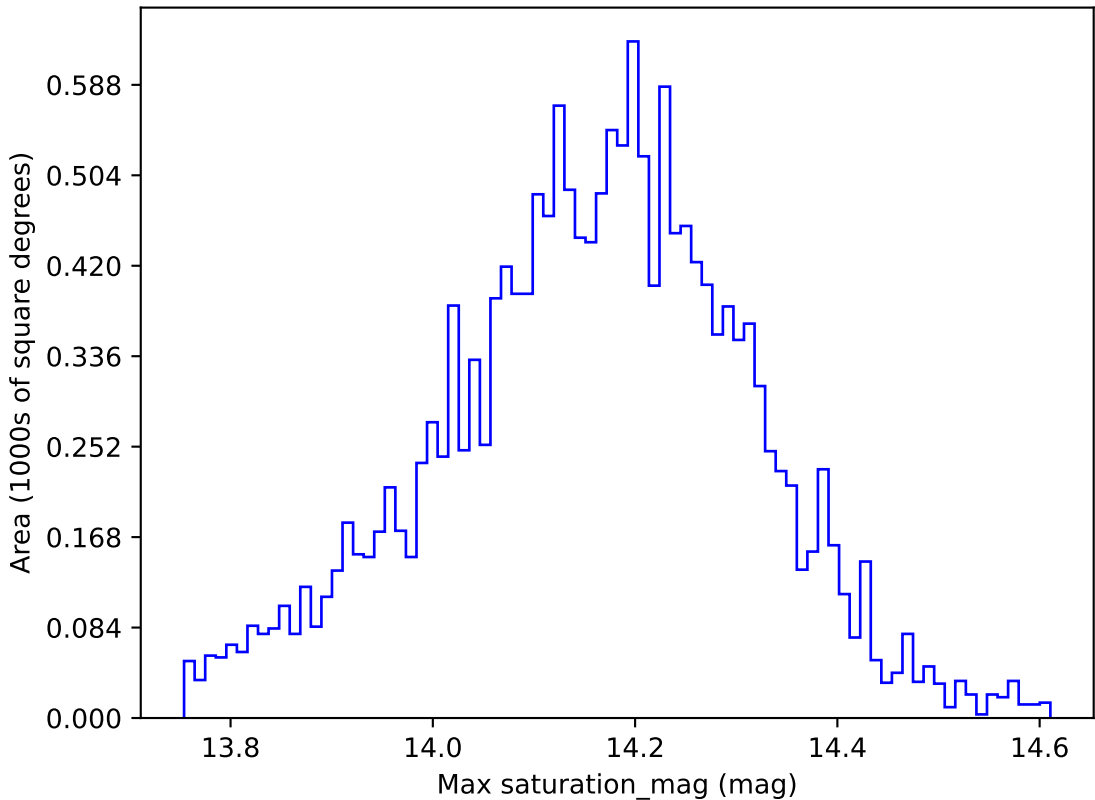
mw_roll_bulge_v3.3_10yrs WFD y band: Max saturation_mag
