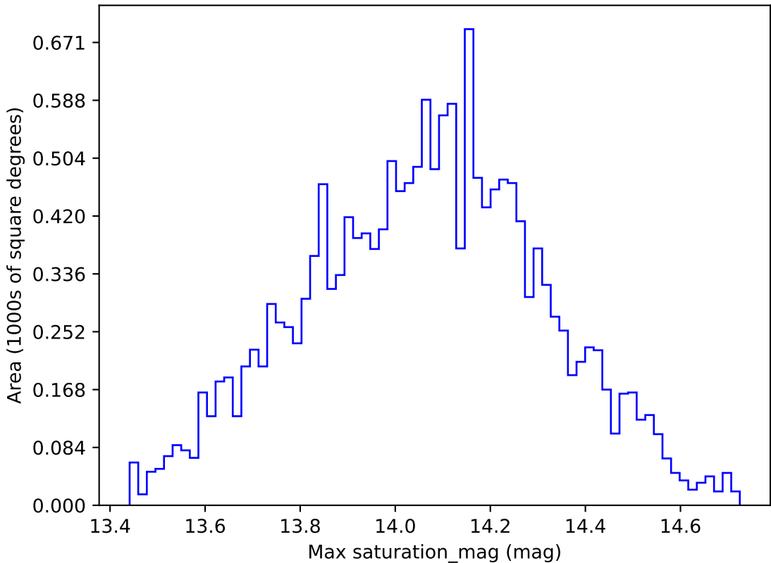
mw_roll_bulge_v3.3_10yrs WFD u band: Max saturation_mag
