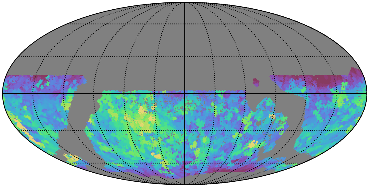
mw_roll_bulge_v3.3_10yrs WFD r band: Max saturation_mag
