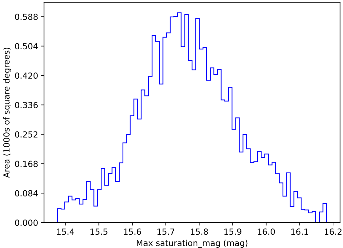
mw_roll_bulge_v3.3_10yrs WFD r band: Max saturation_mag
