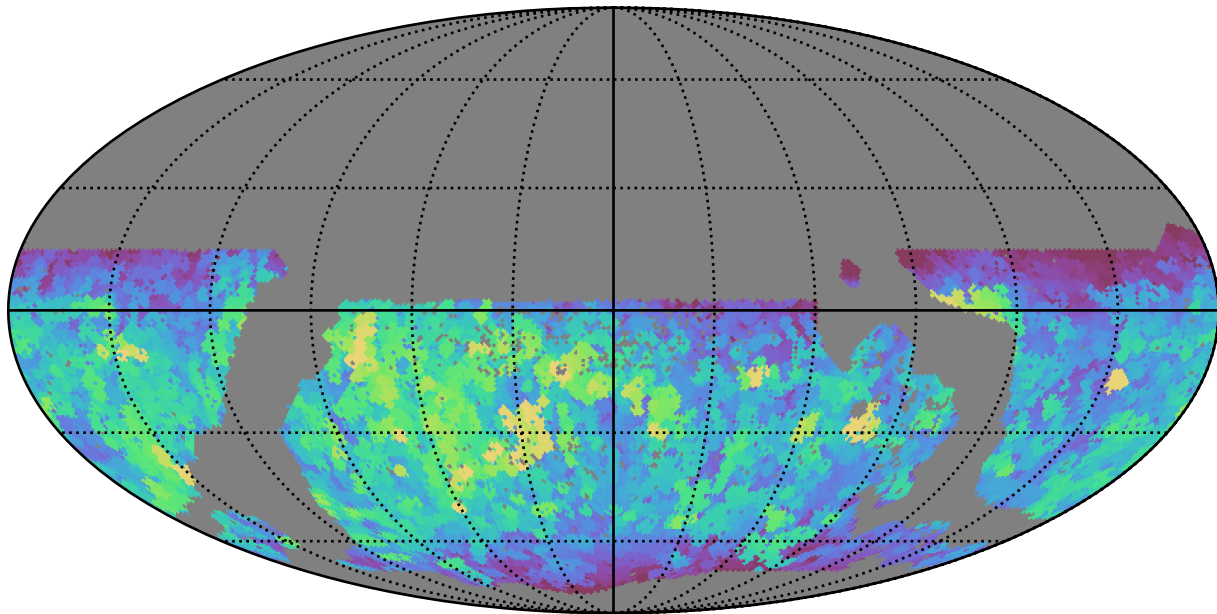
mw_roll_bulge_v3.3_10yrs WFD i band: Max saturation_mag
