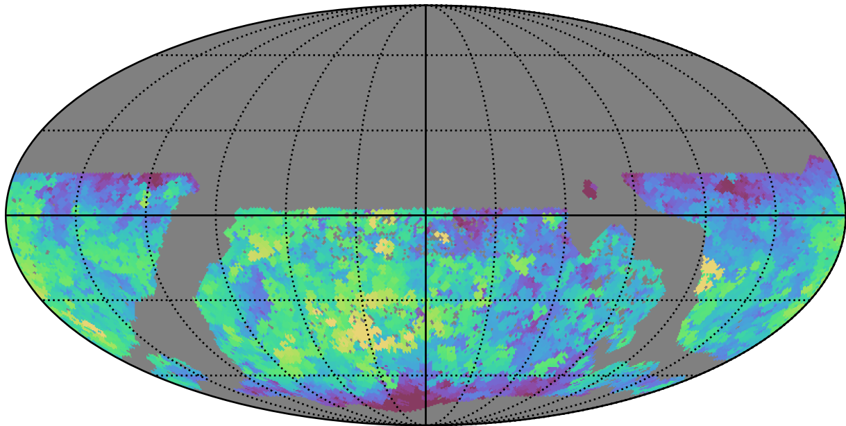
mw_roll_bulge_v3.3_10yrs WFD g band: Max saturation_mag
