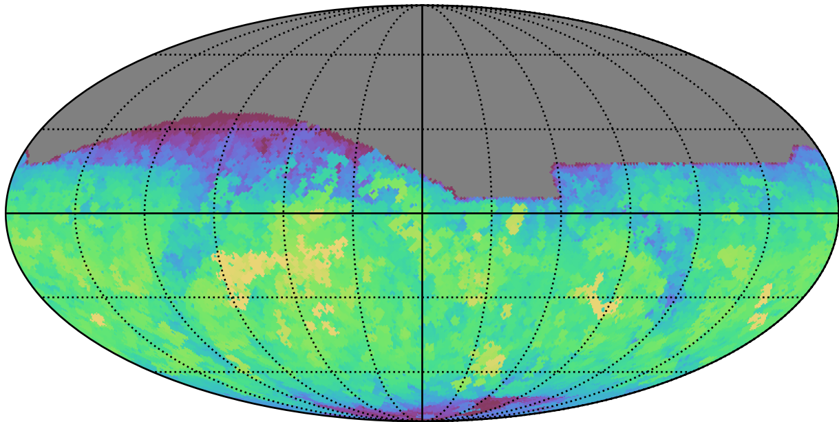
mw_roll_bulge_v3.3_10yrs All sky z band: Max saturation_mag
