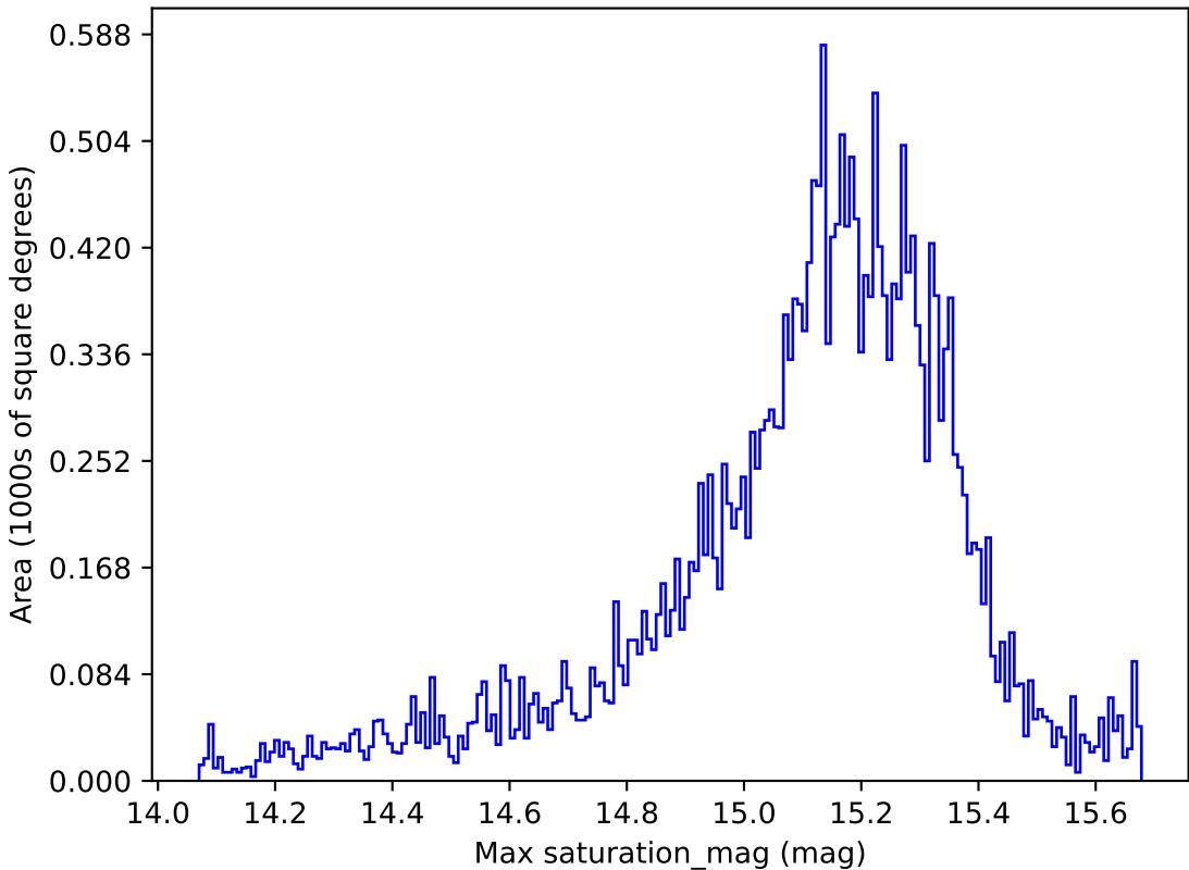
mw_roll_bulge_v3.3_10yrs All sky z band: Max saturation_mag
