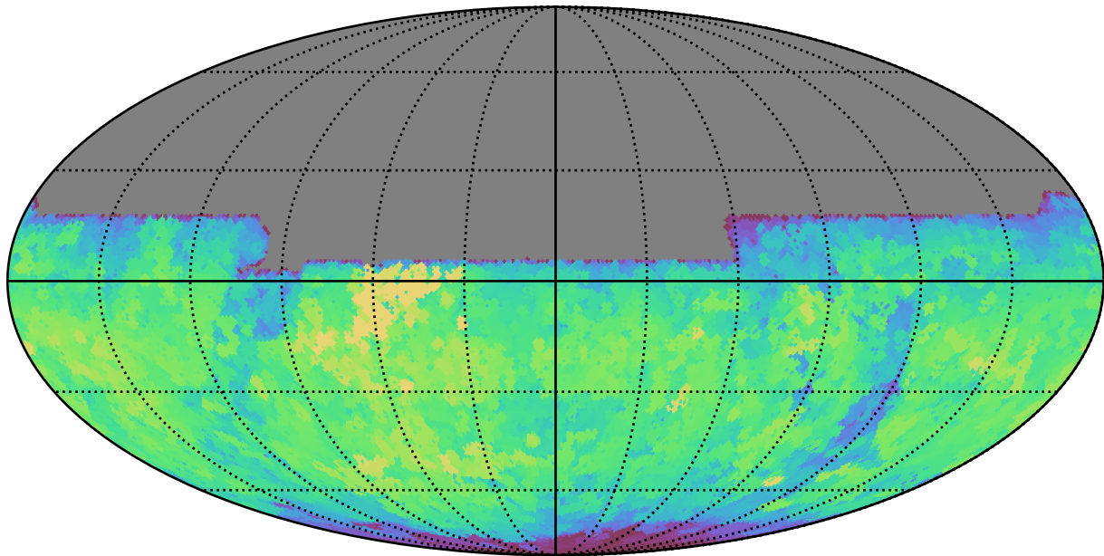
mw_roll_bulge_v3.3_10yrs All sky y band: Max saturation_mag
