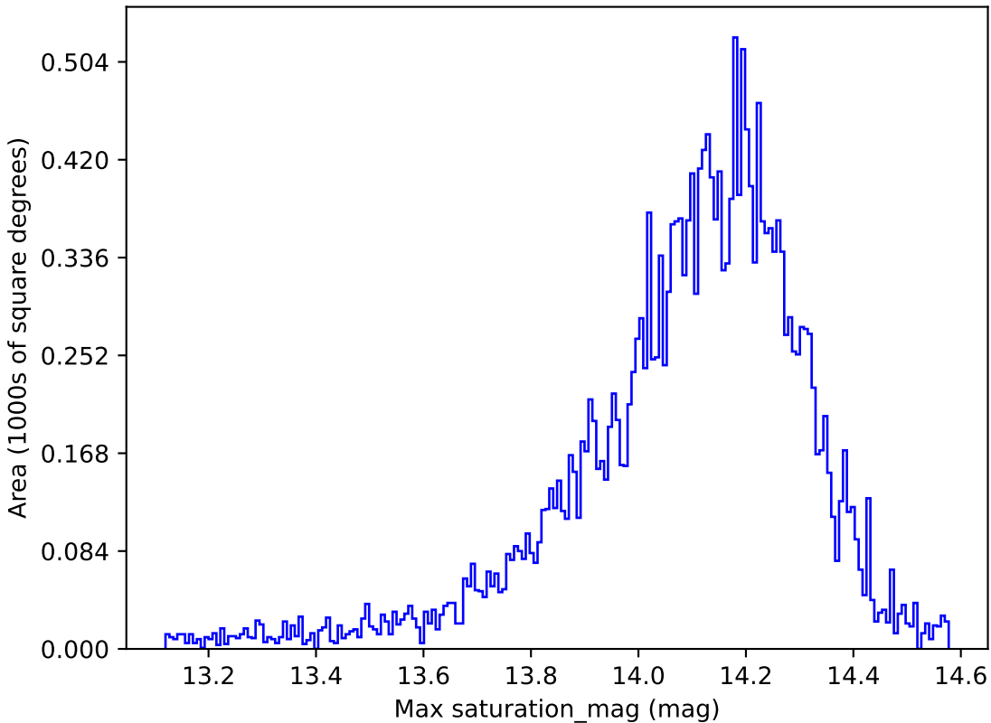
mw_roll_bulge_v3.3_10yrs All sky y band: Max saturation_mag
