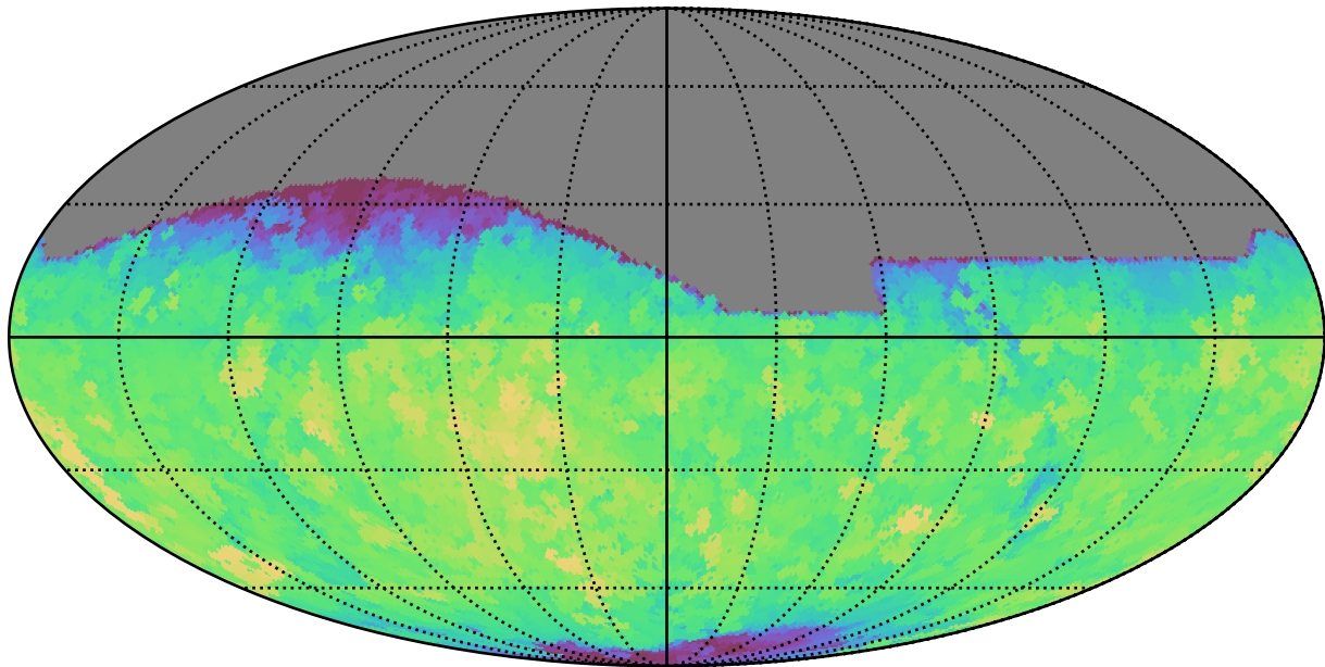
mw_roll_bulge_v3.3_10yrs All sky r band: Max saturation_mag
