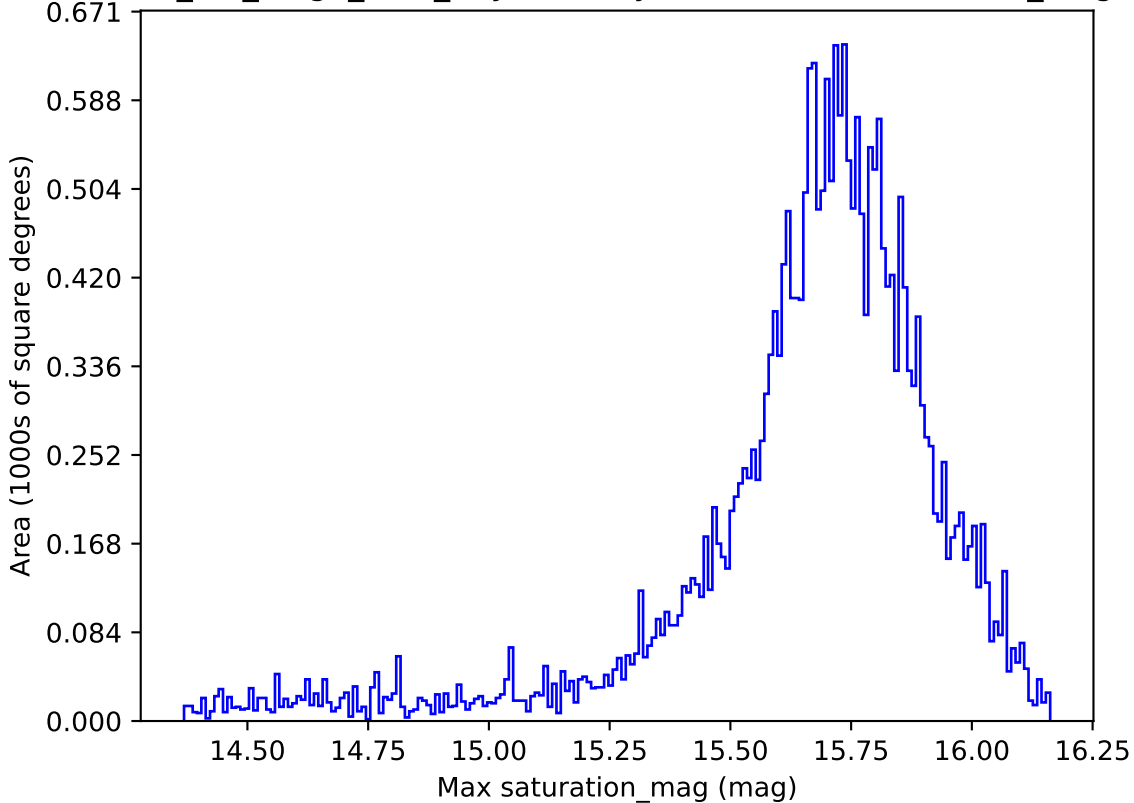
mw_roll_bulge_v3.3_10yrs All sky r band: Max saturation_mag
