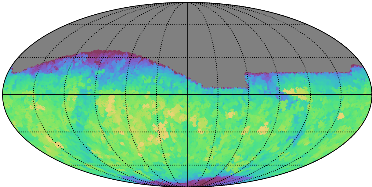
mw_roll_bulge_v3.3_10yrs All sky i band: Max saturation_mag
