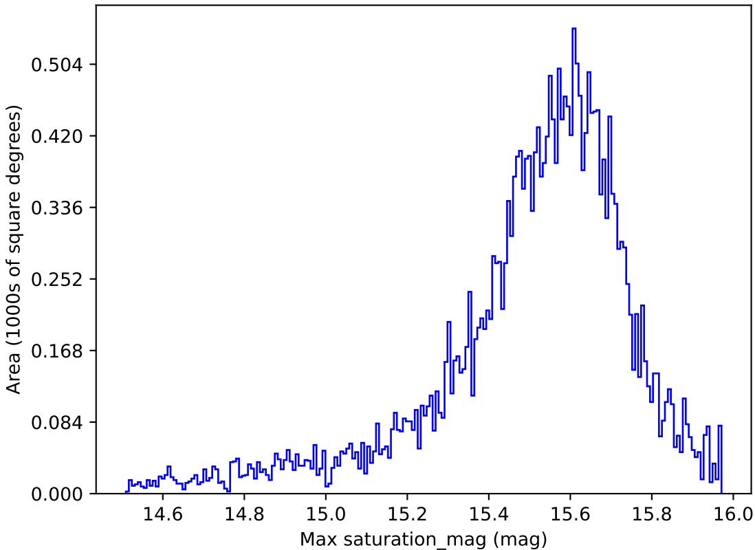
mw_roll_bulge_v3.3_10yrs All sky i band: Max saturation_mag
