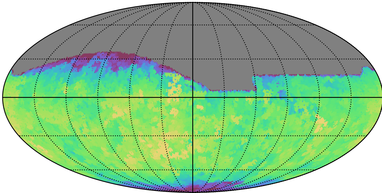
mw_roll_bulge_v3.3_10yrs All sky g band: Max saturation_mag
