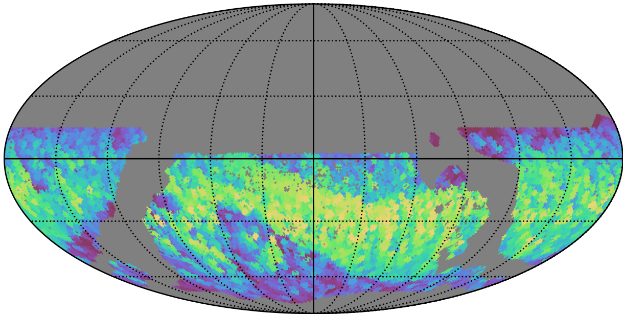
mw_roll_bulge_v3.3_10yrs WFD z band: Max normairmass
