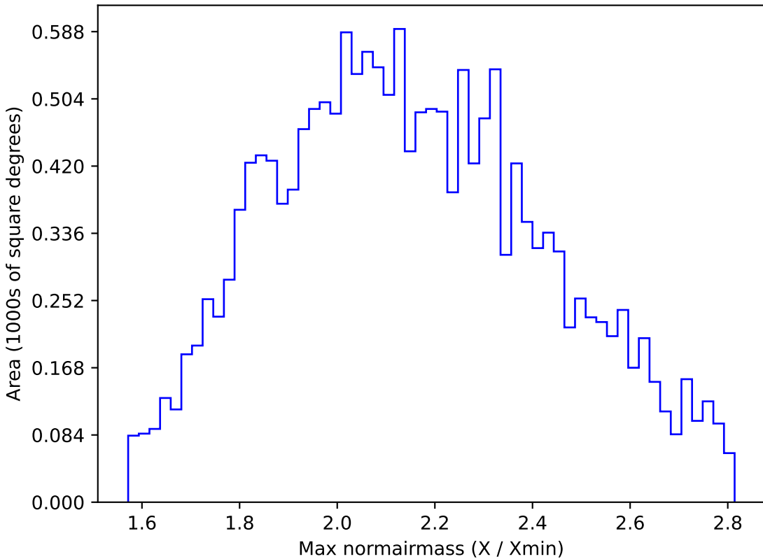
mw_roll_bulge_v3.3_10yrs WFD y band: Max normairmass
